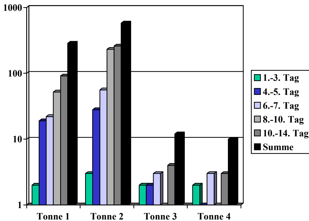
Abb. 2: Darstellung der Anflugaktivität bei einer Standzeit von 14 Tagen
